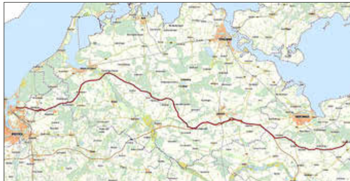
Verlauf der HYROW-Wasserstoff-Pipeline
