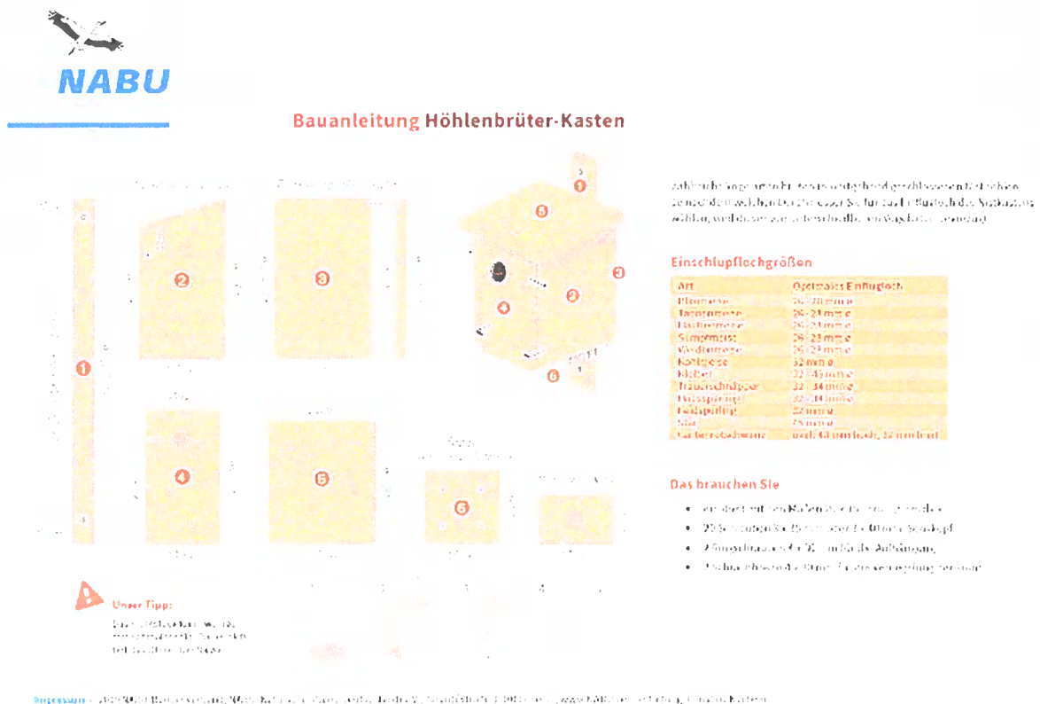
Abb. 8: Höhlenbrüter – Nistkasten (Quelle © NABU)
